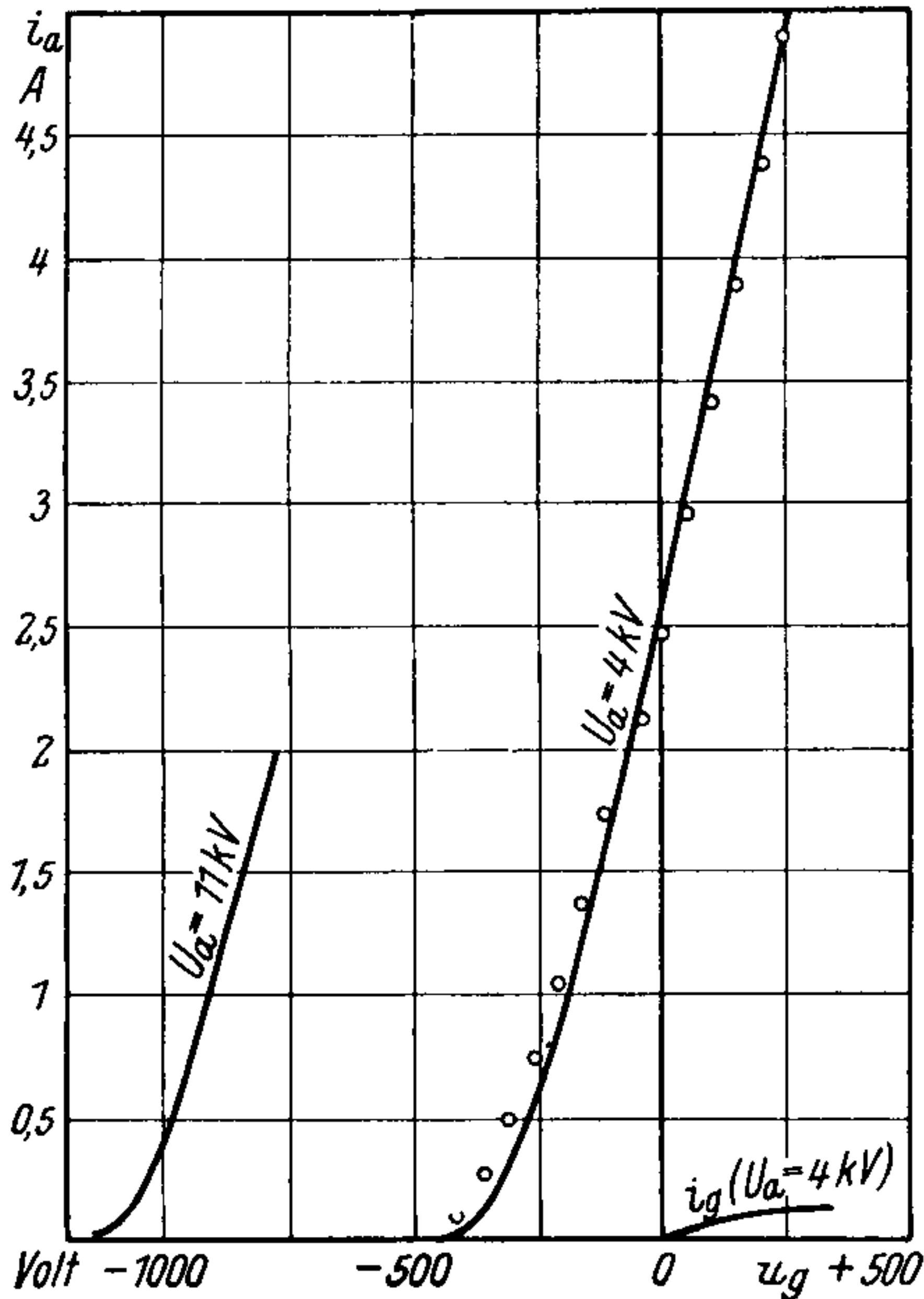
Bild 16. Statische Kennlinien der Telefunkenröhre RS 261.
