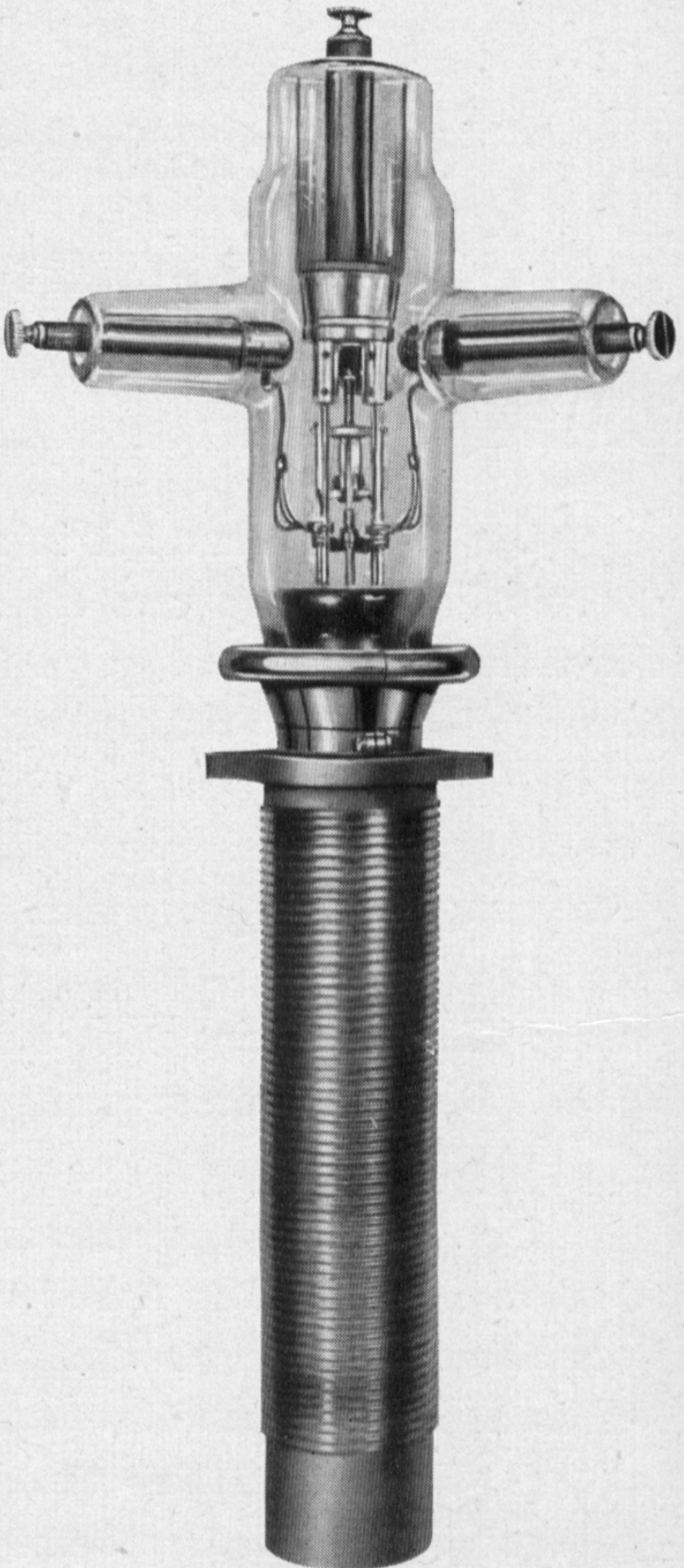
Bild 17. 10-kW-Modulatorröhre RS 261 (Telefunken).
