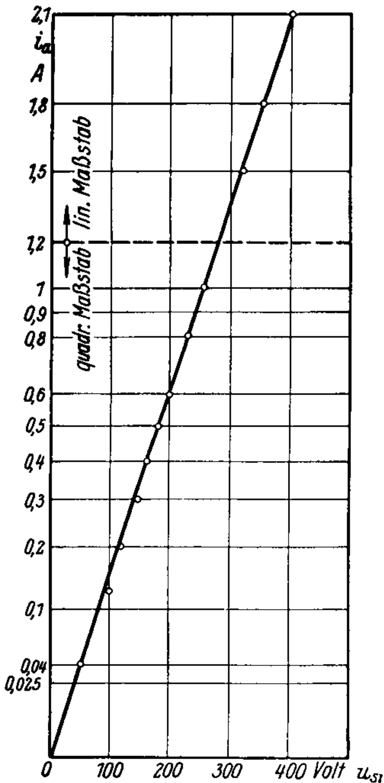
Bild 18. Statische Kennlinie der RS 261 mit teils quadratischem, teils linearem i_a -Maßstab.
